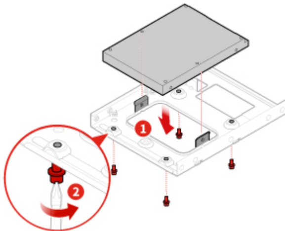
Abbildung 39. Neues primäres 2,5-Zoll-Speicherlaufwerk in den Speicherkonverter installieren
