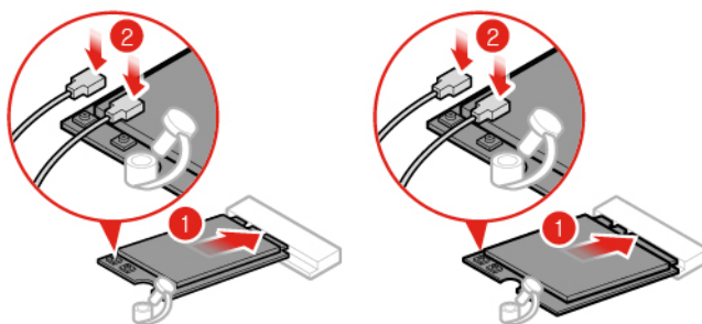
Abbildung 60. Wi-Fi-Karte installieren und Wi-Fi-Antennen (Typ 1 und Typ 2) anschließen
