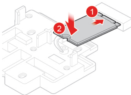
Abbildung 75. M.2-Solid-State-Laufwerk installieren
