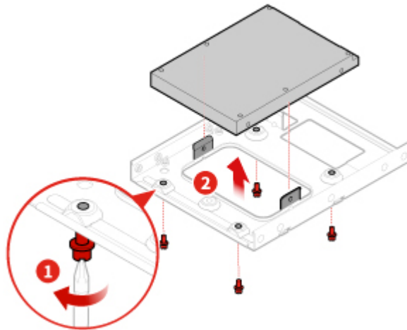
Abbildung 38. Primäres 2,5-Zoll-Speicherlaufwerk aus dem Speicherkonverter entfernen
