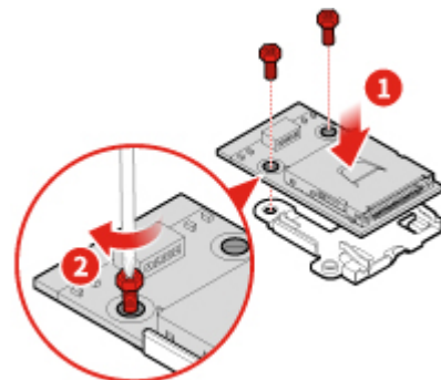
Abbildung 109. Platine des Leseegeräts für Speicherkarten installieren
