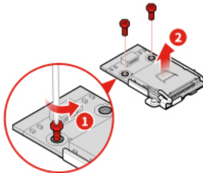
Abbildung 108. Platine des Leseegeräts für Speicherkarten entfernen
