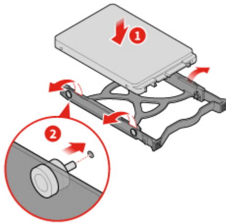
Abbildung 44. Die Blende für das sekundäre 2,5-Zoll-Speicherlaufwerk installieren
