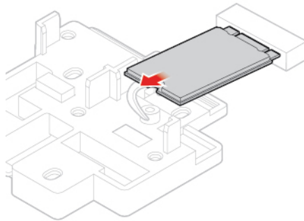
Abbildung 74. M.2-Solid-State-Laufwerk entfernen
