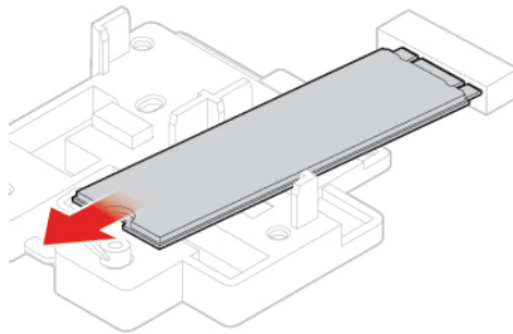
Abbildung 66. M.2-Solid-State-Laufwerk entfernen
