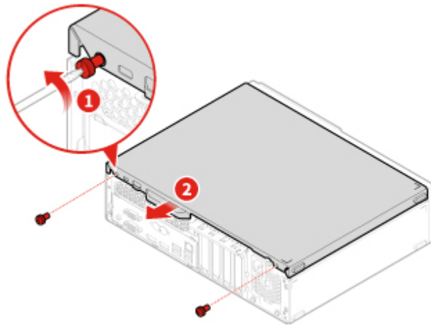
Abbildung 25. Computerabdeckung entfernen
