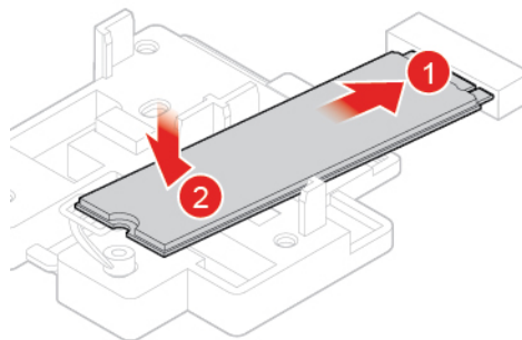
Abbildung 67. M.2-Solid-State-Laufwerk installieren
