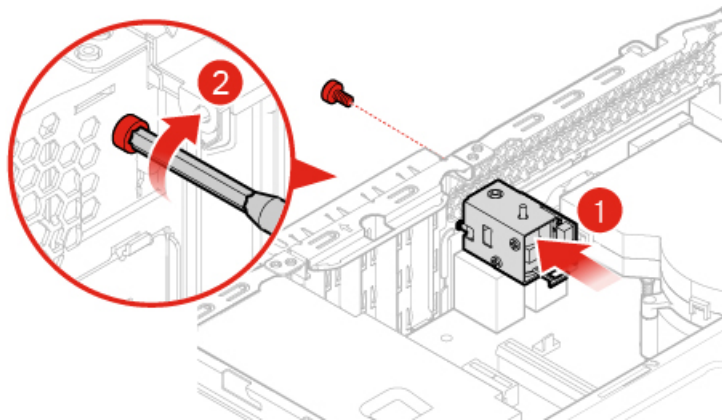
Abbildung 128. E-Schloss installieren
