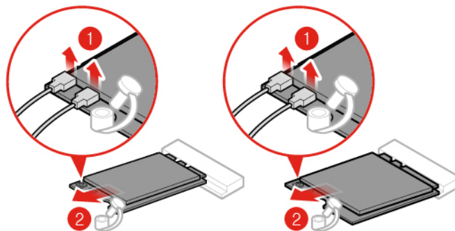
Abbildung 59. Wi-Fi-Antennen abziehen und Wi-Fi-Karte (Typ 1 und Typ 2) entfernen
